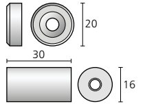
kit B 30 Ø 20 x d 6 - Ø 16 x d 30mm Ø 0,79 x d 0,24" - Ø 0,63 x d 1,18"
