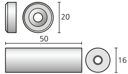
kit B 50 Ø 20 x d 6 - Ø 16 x d 50mm Ø 0,79 x d 0,24" - Ø 0,63 x d 1,97"
